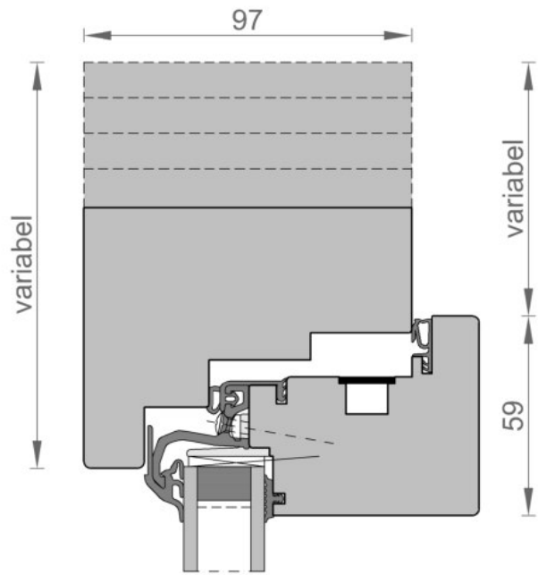
Integralfenster
