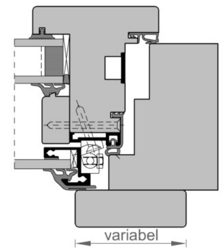
Verbundfenster
