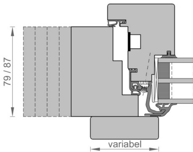
Integralfenster
