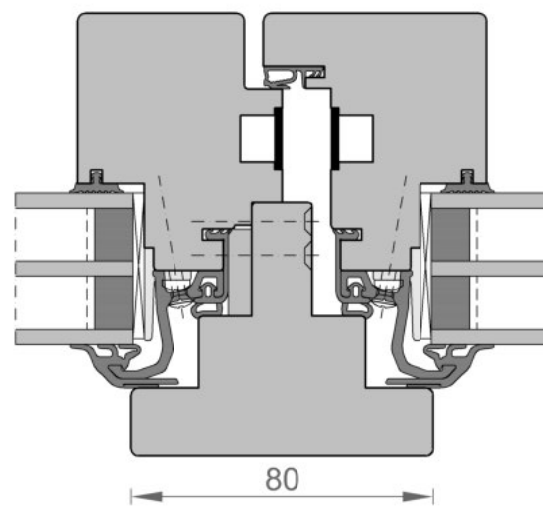
Stulpfenster
