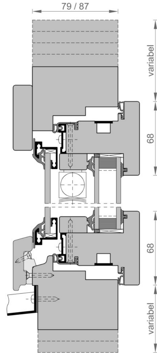
Verbundfenster
