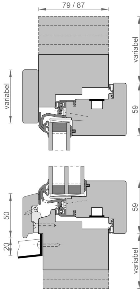
Integralfenster
