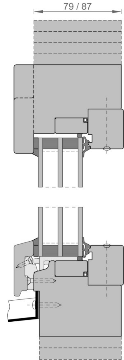
Festverglasung
